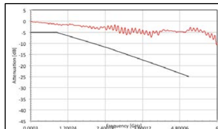
18Ghz Attenuation
